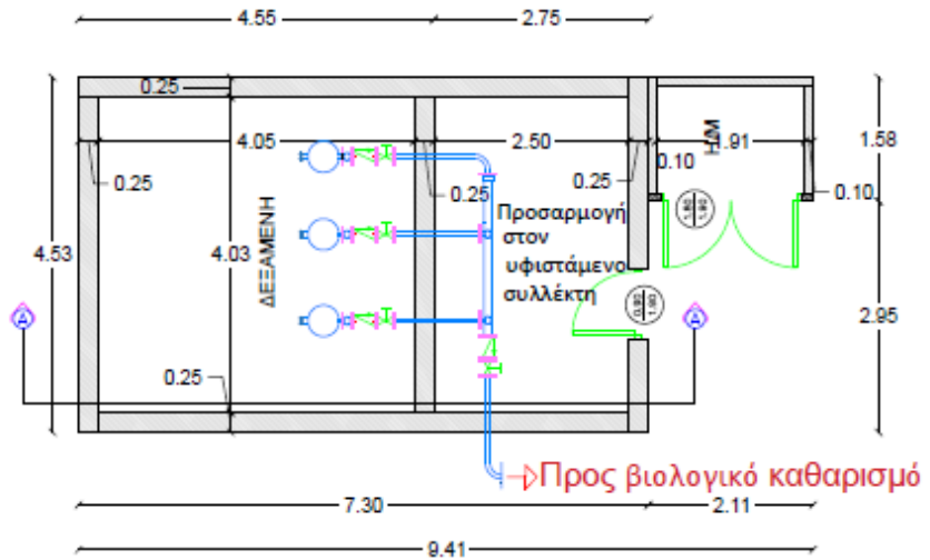
Κάτοψη υφιστάμενης δεξαμενής – αντλιοστασίου λυμάτων
