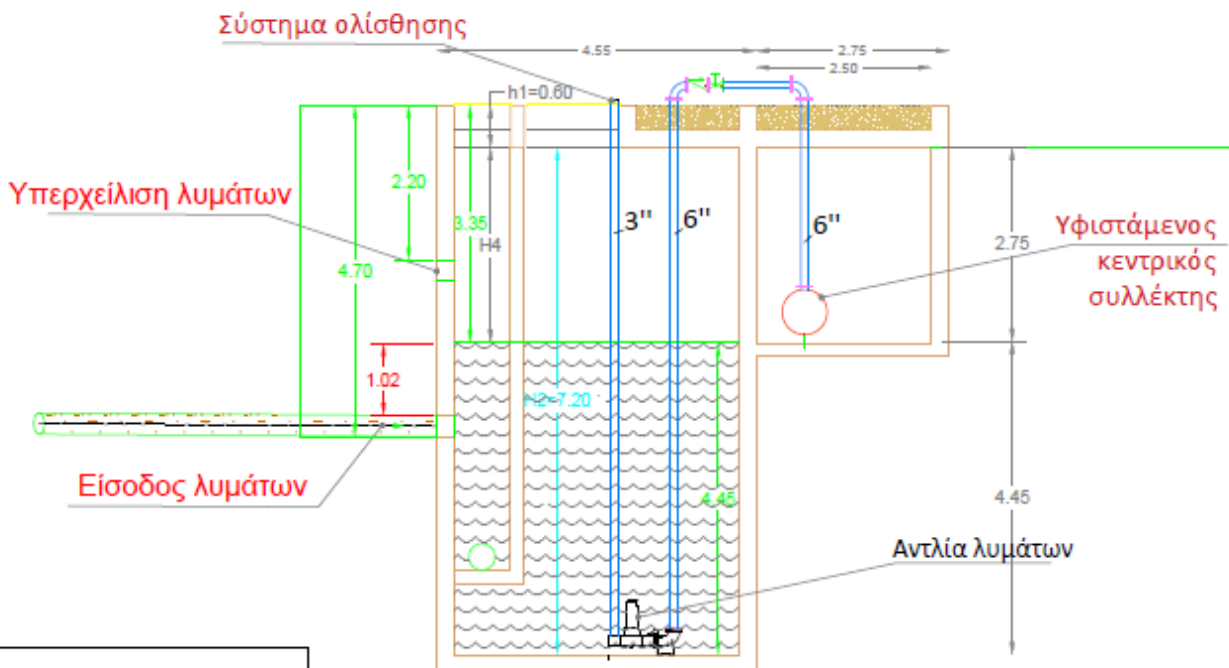
Τομή ΑΑ υφιστάμενης δεξαμενής – αντλιοστασίου λυμάτων
