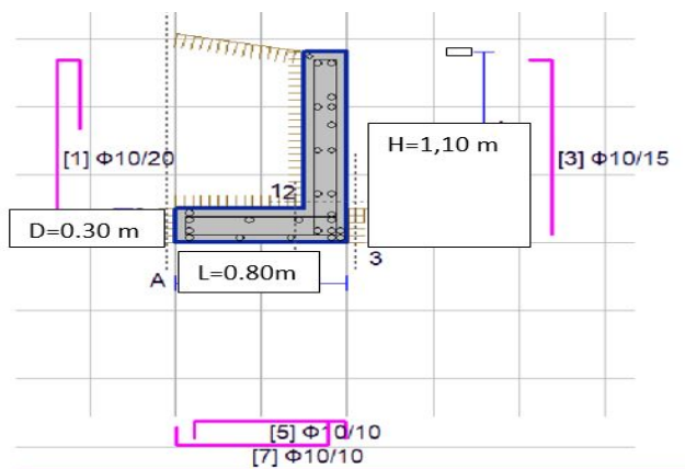
ΣΧ 2. Διατομή τοιχίου
