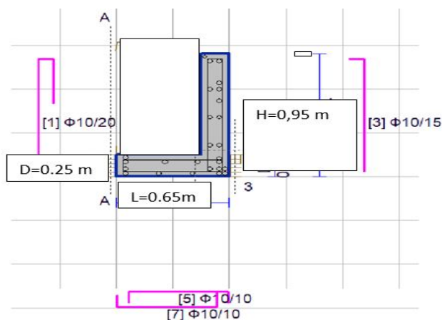
ΣΧ 3. Διατομή τοιχίου
